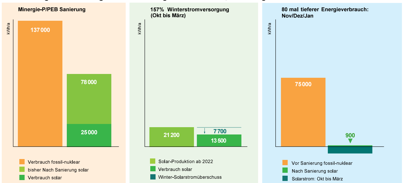
4 157%-Winterstromversorgung: Der Winter-Solarstromüberschuss von 7'700 kWh ersetzt die im Nov./Dez./Jan. fehlenden 900 kWh noch im Winter über 8 mal.
